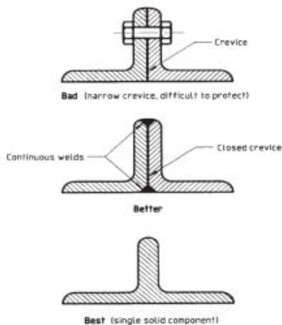
图 D.3 - 缝隙的处理
